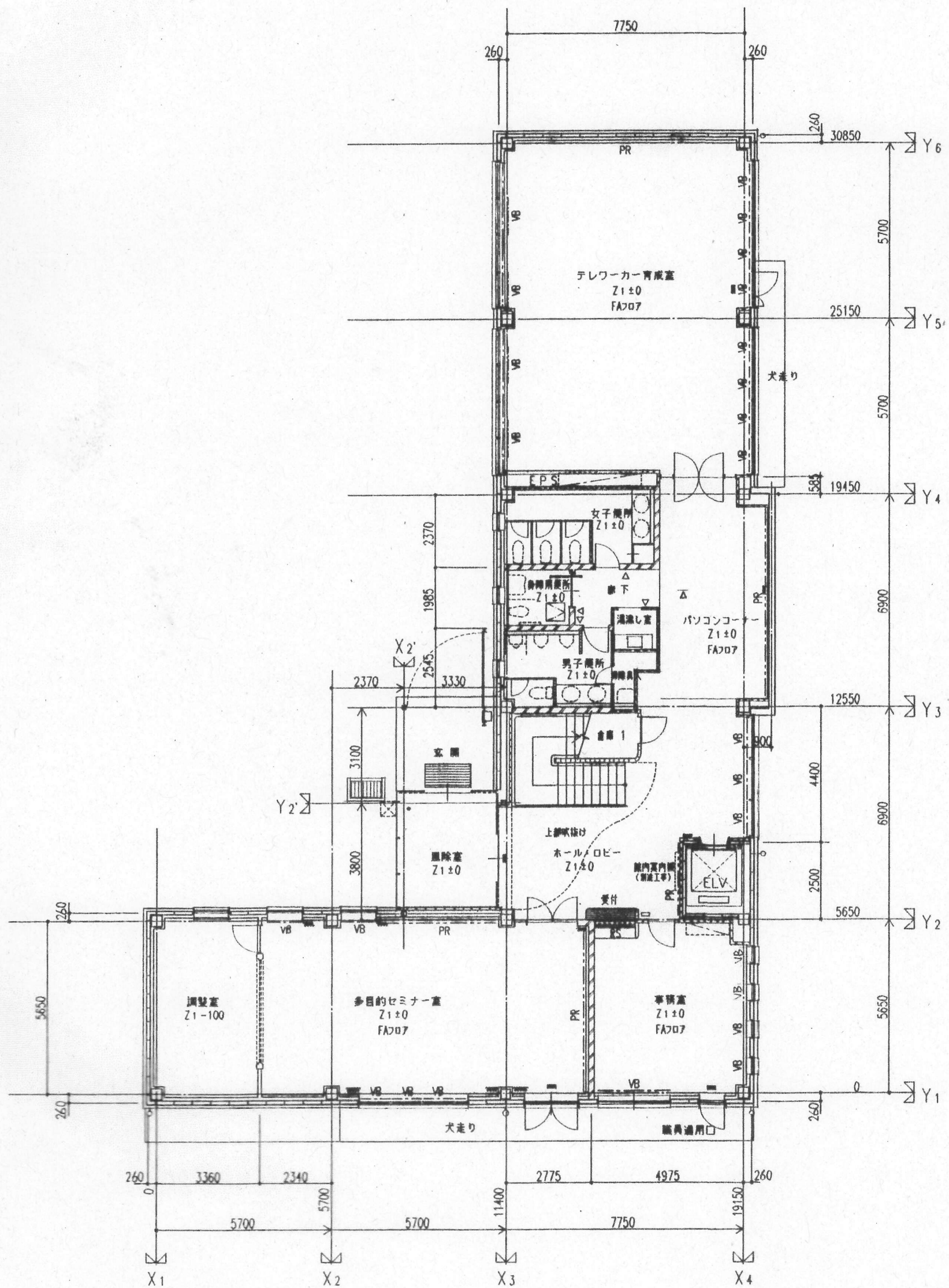
Z1 平面図
