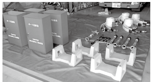
▲消火栓放水器具一式
