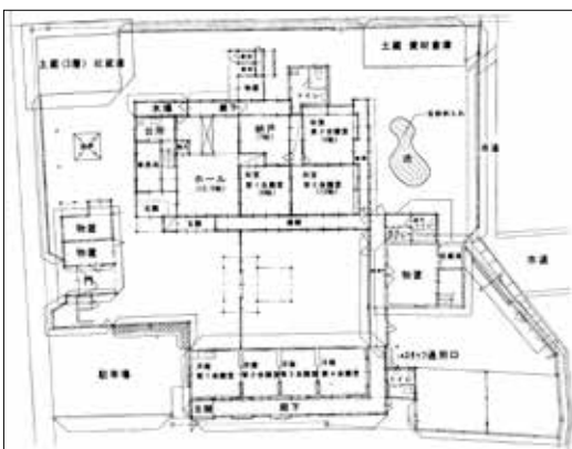
▲施設平面図
