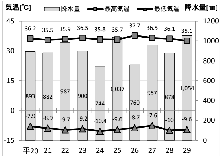
■土地面積の割合(平成30年(2018年)1月1日現在) ■気温(最高・最低)と降水量の推移 (資料)税務課 (資料)長野地方気象台、須坂建設事務所
