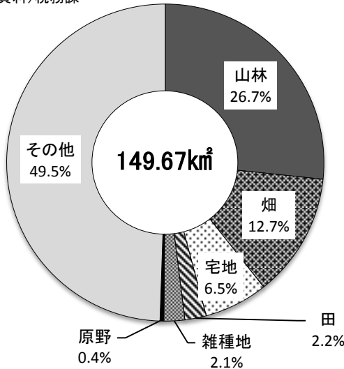
■土地面積の割合(平成30年(2018年)1月1日現在) ■気温(最高・最低)と降水量の推移 (資料)税務課 (資料)長野地方気象台、須坂建設事務所
