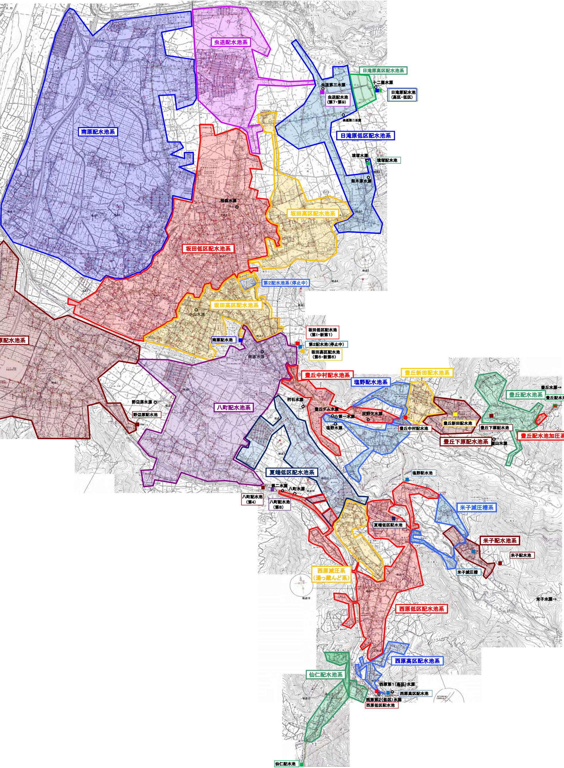
須坂市配水池系全体図
